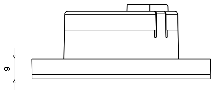
Vista da destra Scala: 1:1
