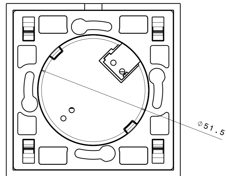
Vista dal basso Scala: 1:1
