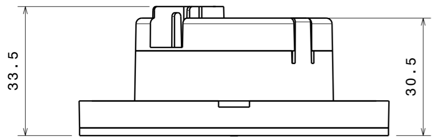
Vista da sinistra Scala: 1:1
